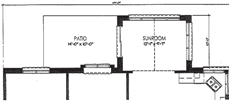
OPTIONAL SUNROOM PLAN
