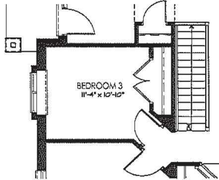
OPTIONAL BEDROOM 3 PLAN
